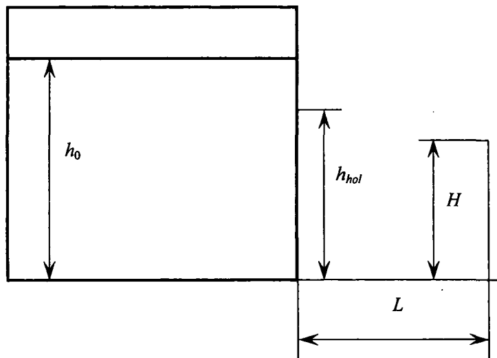
Рис. П3.1. Схема для расчета истечения жидкости из отверстия в резервуаре
